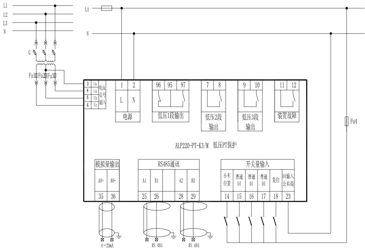
图 7 三相三线、强电开入
