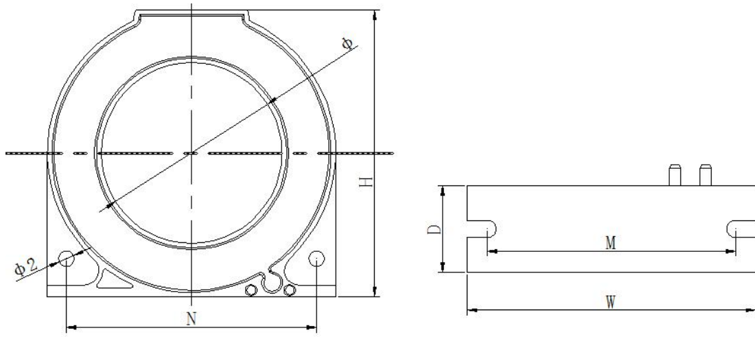
互感器部分
